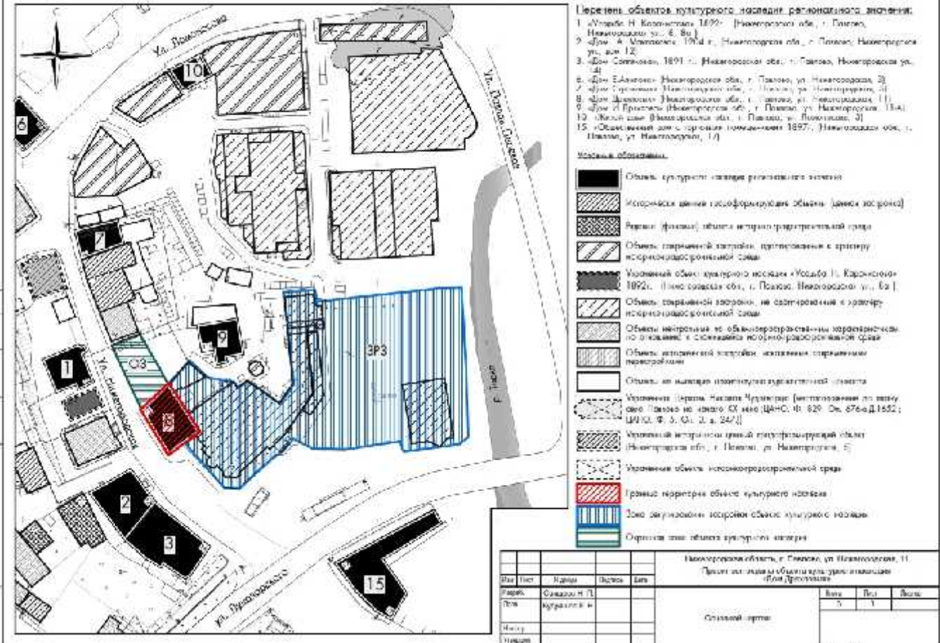
Проект зон охраны объекта культурного наследия «Дом Давыдова», ул. Нижегородская, 11. Основной чертеж.
